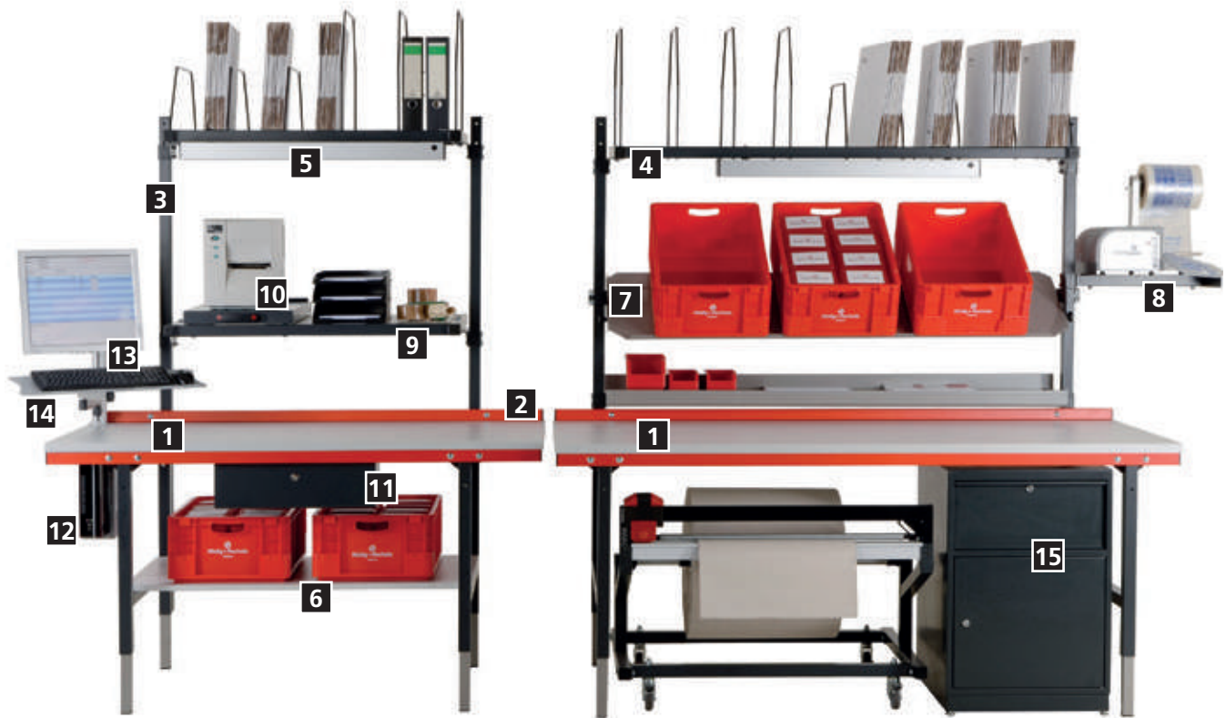
Zubehör für die Tischbreite 1600 und 2000 mm
