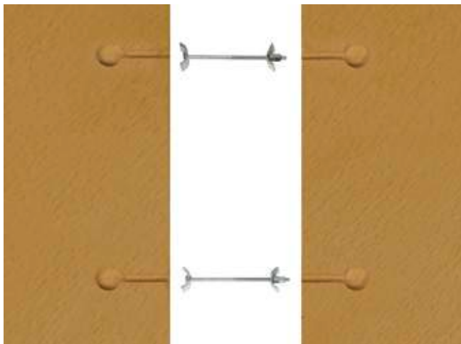
Platte - Platte - Verbinder ■ Mit Lamello und 2 Spannklemmern ■ Für Längen ab 2500 mm
