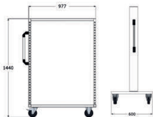
Multi-Wagen ■ Unbestückt
