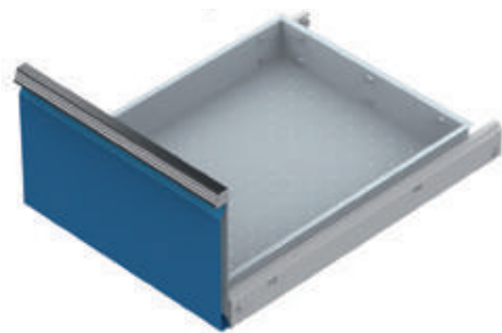
Schubladen CNC Breite 600 x 600 mit Vollauszug 100 % - 180 kg
